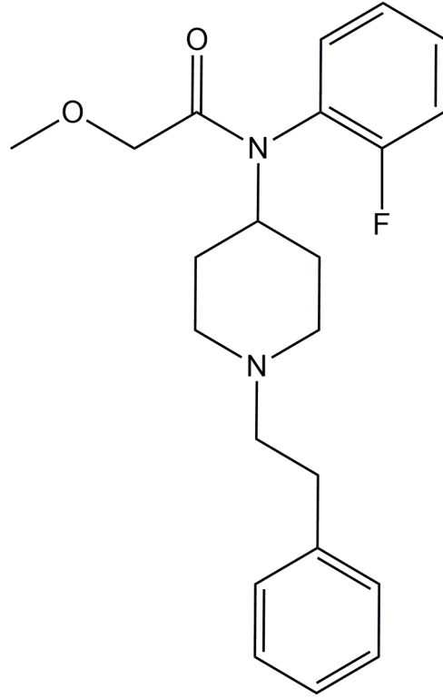
Ocfentanil
